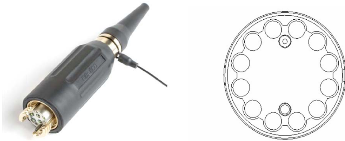
Bild 4.15: Linsenstecker von Fibreco und Draufsicht
