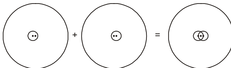
Bild 4.3: Kern-Mantel-Exzentrizität
